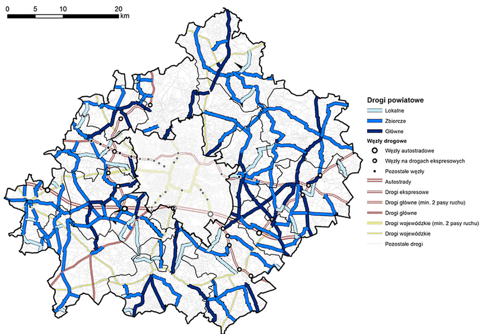
Ryc. 4. Sieć dróg powiatowych z podziałem na klasy techniczne
