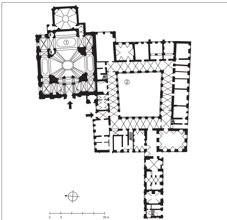
Owińska, dawny zespół klasztorny cysterek. Przekrój poziomy parteru. 1 – kościół, obecnie parafialny; 2 – klasztor, obecnie Specjalny Ośrodek Szkolno-Wychowawczy dla Dzieci Niewidomych w Owińskich
