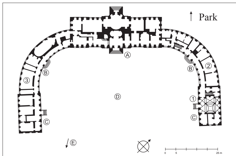
Pałac w Rogalinie. Przekrój poziomy parteru.
